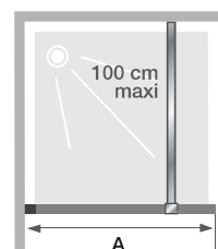
Installation réversible gauche / droite
